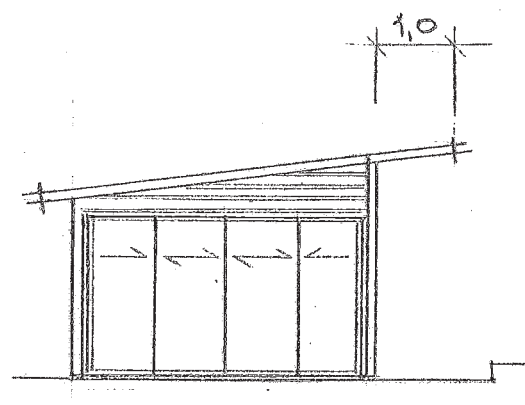
FASAD MOT SÖDER, 1:100
